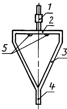
Маятник А
