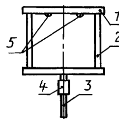
Маятник Б
