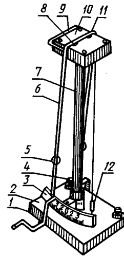
1 — пусковой механизм; 2 — основание; 3 — шкала; 4 — установочные винты; 5 — груз; 6 — двустрелочный маятник; 7 — штатив; 8 — соединительная планка; 9 — рамка; 10 — столик; 11 — стальные шарики; 12 — отвес
